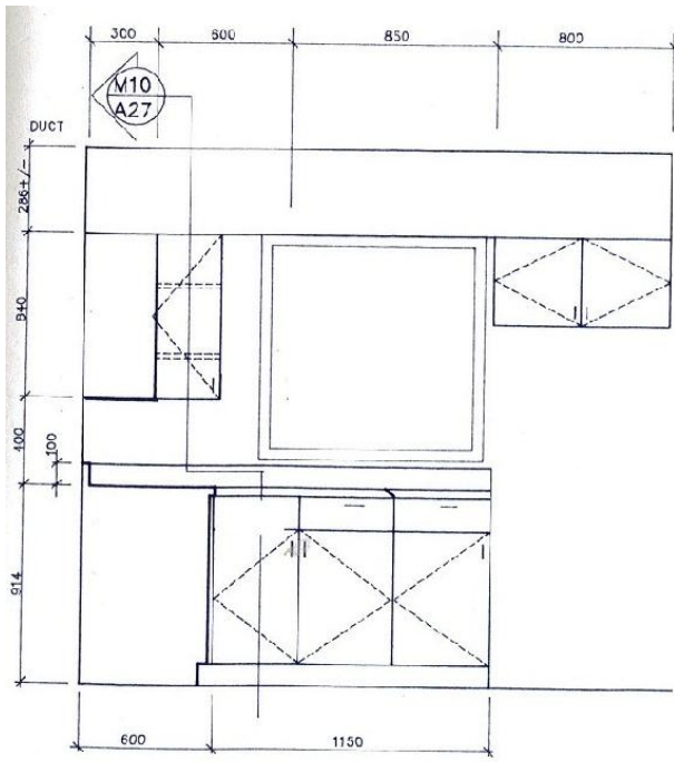
ELEVATION
